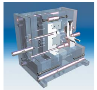
Kompletna forma wtryskowa zbudowana z elementów znormalizowanych HASCO
